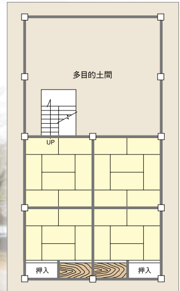
幸喜山荘 間取図(1階)
