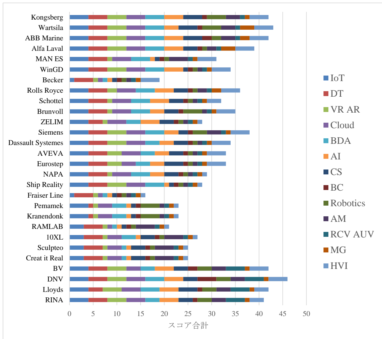
図表 5：欧州の船用機器メーカー及びソリューション提供企業のデジタルトランスフォーメーションスコア
