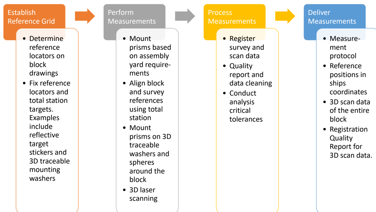
図表 7: 3D データ記録プロセスの概要
