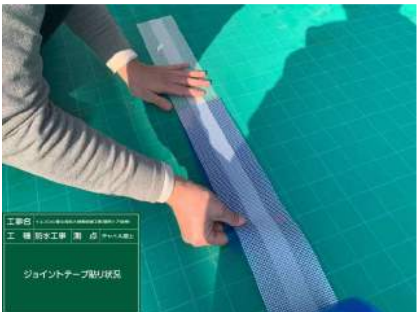
工事名 千葉県庁庁舎の屋根防水工事 工 種 防水工事 測 点 チャペル屋上 ジョイントテープ貼り状況
