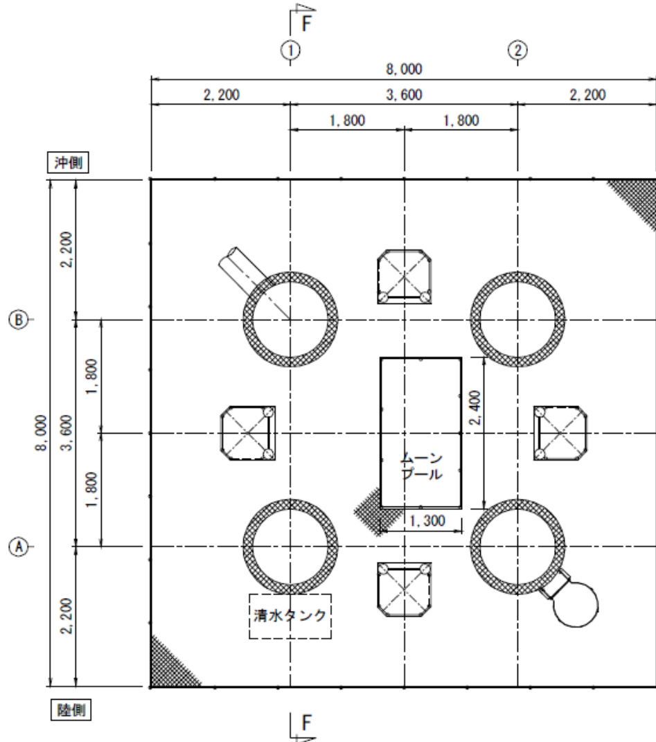
Platform lower deck 平面図 (C-C平面図)
