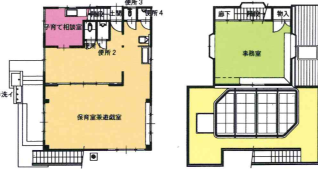
保育所棟1階平面図
