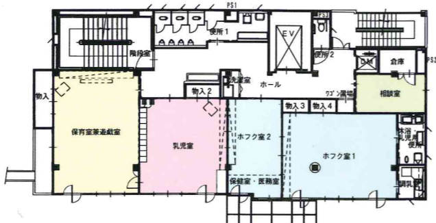
複合施設棟2階平面図
