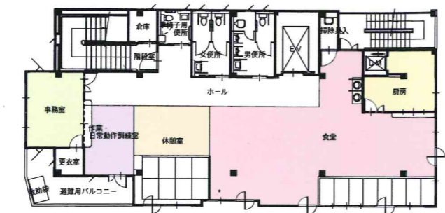
複合施設棟3階平面図
