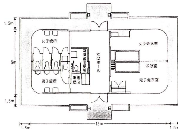
クラブハウス 平面図
