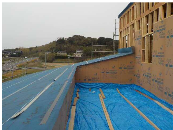
断熱材施工工事
