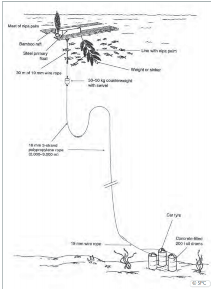
図 VI-9 パヤオのシステム
