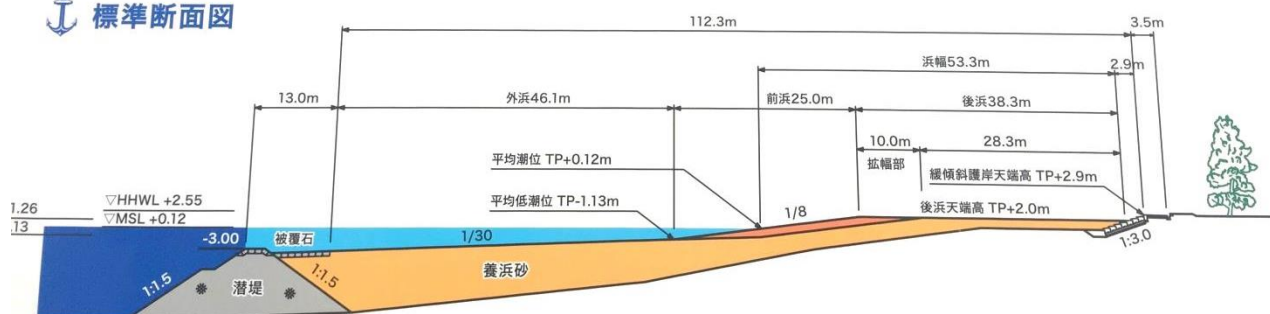
標準断面図
