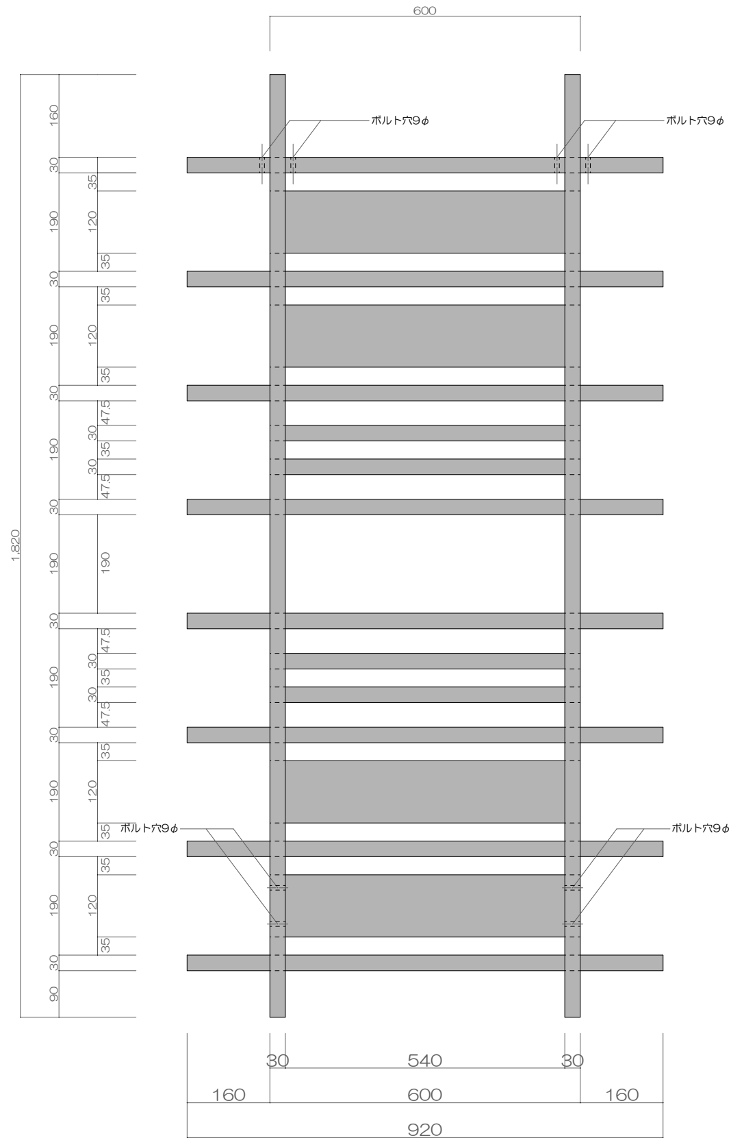
正面図
