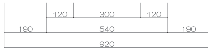
正面図
