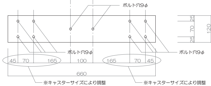
上面図
