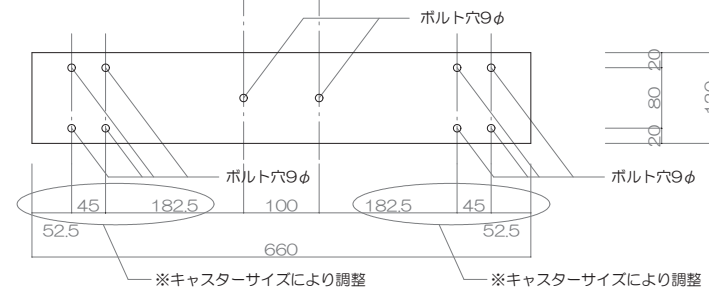
上面図
