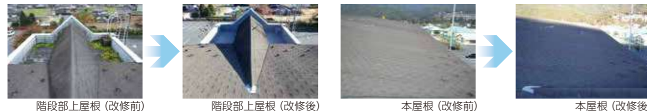
階段部上屋根(改修前) 階段部上屋根(改修後) 本屋根(改修前) 本屋根(改修後)
