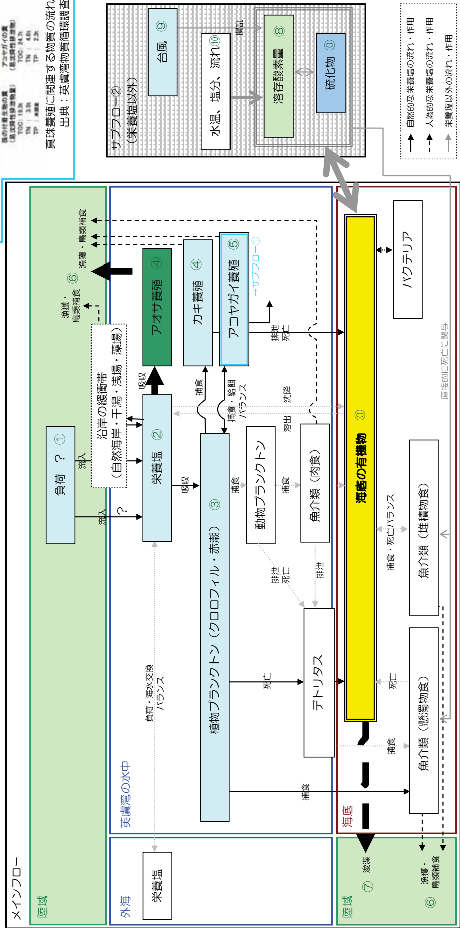
図 3.19 かつてと現在の物質循環フローの比較 (イメージ)
