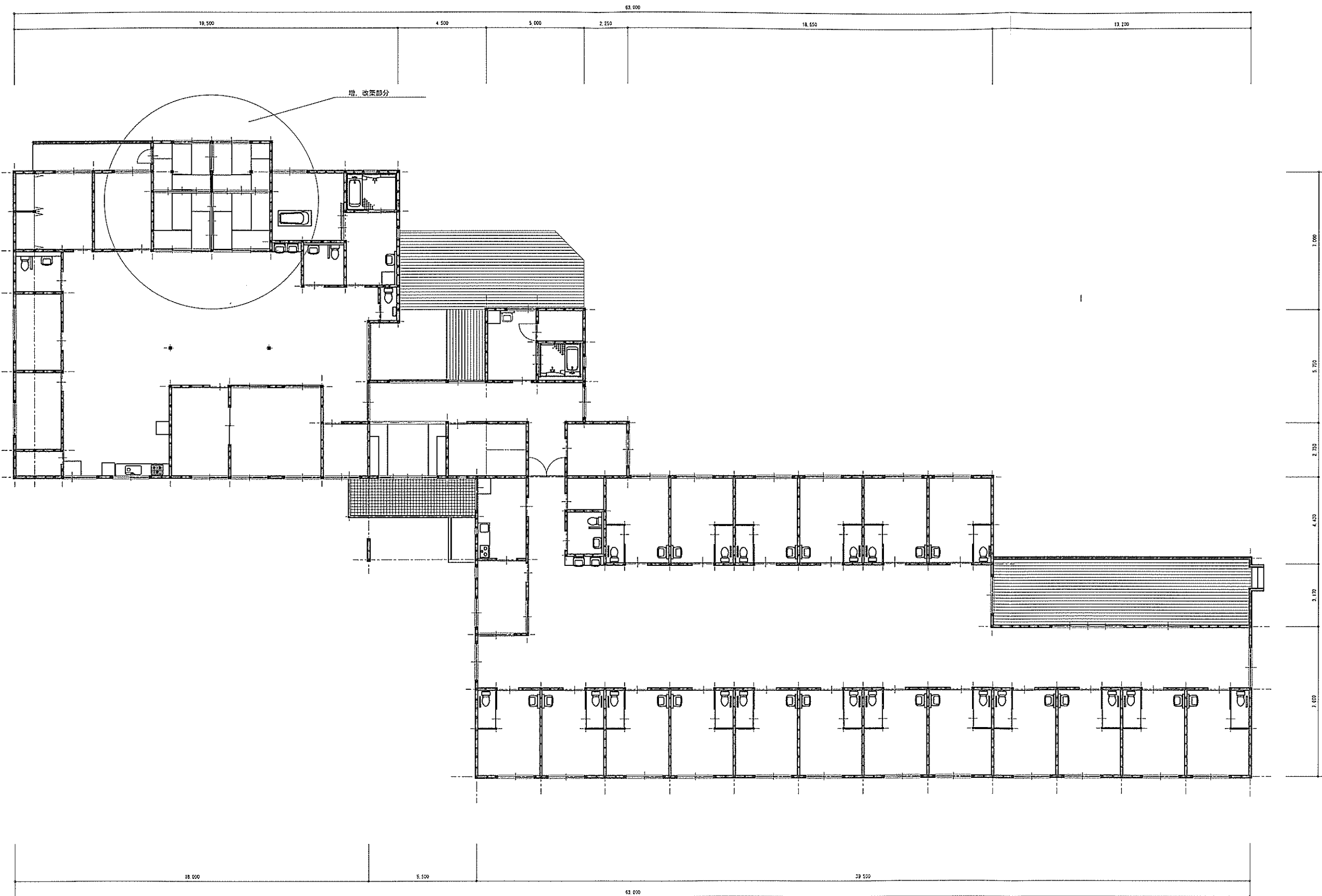
改築後平面図 S = 1 / 100
