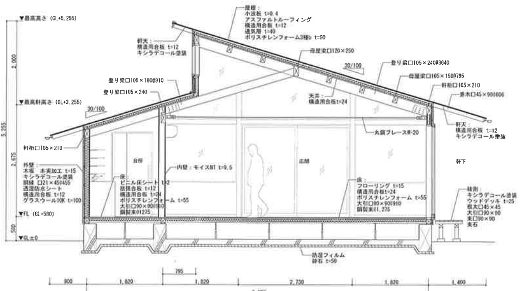
—標準矩計図—
