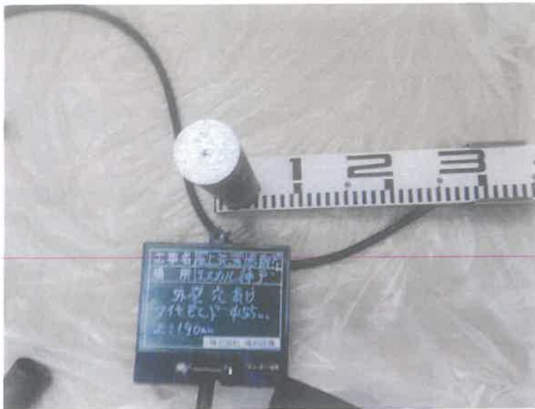
【工事種目】エスカル神戸洗濯給水配管 【施工内容1】屋上外部 【施工内容2】外壁ダイヤモンド貫通 【施工内容3】55mm貫通
