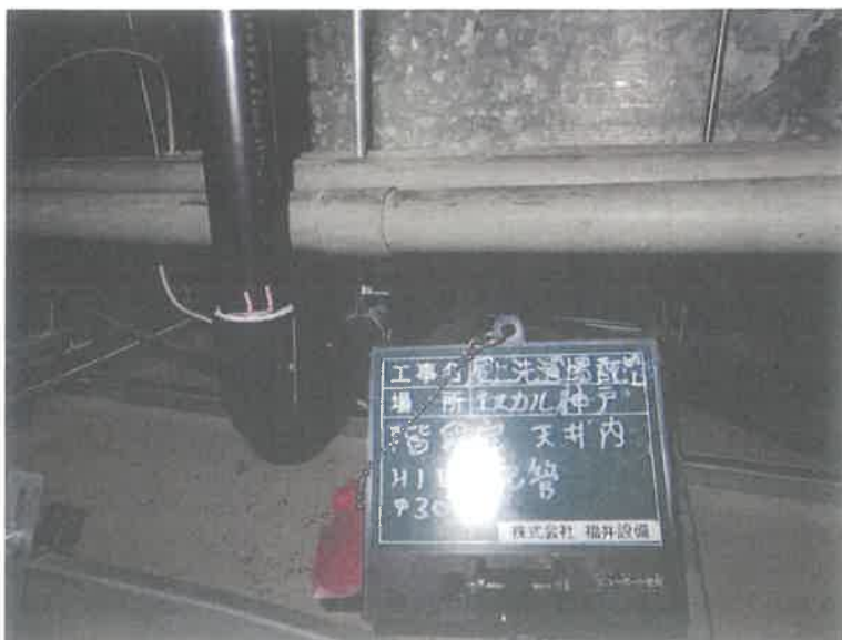
【工事種目】エスカル神戸洗濯給水配管 【施工内容1】5階廊下天井内 【施工内容2】配管作業HIVP30A 【施工内容3】支持金具取付
