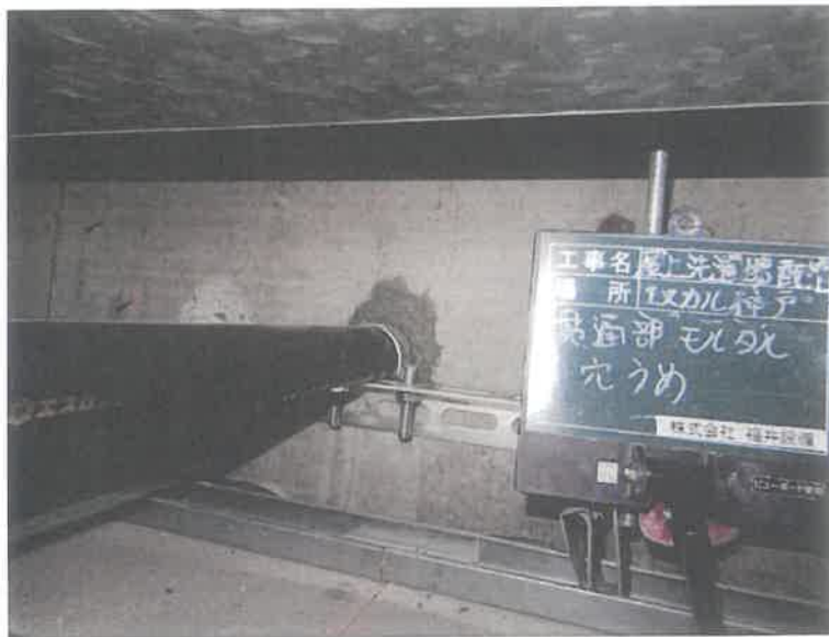
【工事種目】エスカル神戸洗濯給水配管 【施工内容 1】貫通部処理
