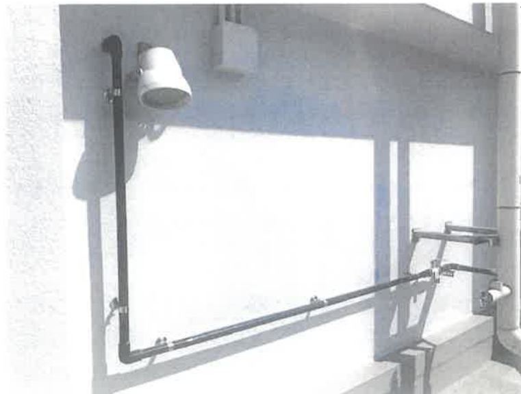
【工事種目】エスカル神戸洗濯給水配管 【施工内容1】屋上外部 【施工内容2】配管作業HIVP30A
