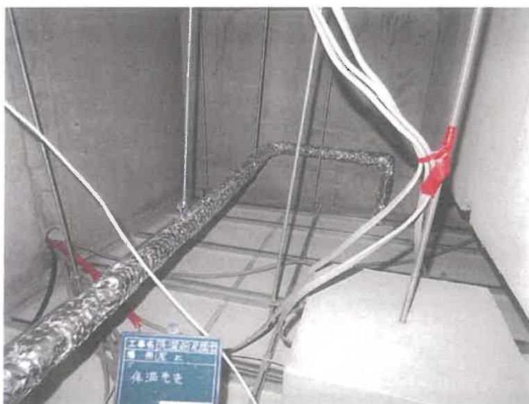
【工事種目】エスカル神戸洗濯給水配管 【施工内容1】5階洗濯室 【施工内容2】室内天井隠蔽部 【施工内容3】グラスウール保温帯/きつ甲金網
