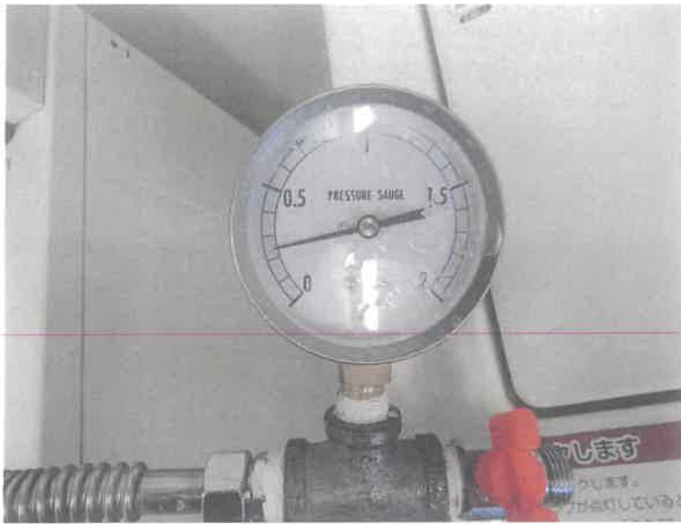
【工事種目】エスカル神戸洗濯給水配管 【施工内容1】5階洗濯室 【施工内容2】切替後水圧測定 【施工内容3】2.5Mpa
