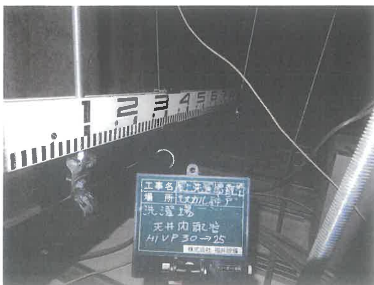
【工事種目】エスカル神戸洗濯給水配管 【施工内容1】5階洗濯室天井内 【施工内容2】配管作業H1VP30A~25A 【施工内容3】支持金具取付
