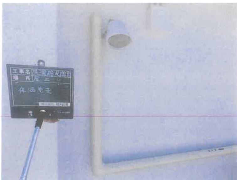
【工事種目】エスカル神戸洗濯給水配管 【施工内容1】5階洗濯室 【施工内容2】屋上外部 【施工内容3】ポリスチレンフォーム保温筒/カラー亜鉛鉄板
