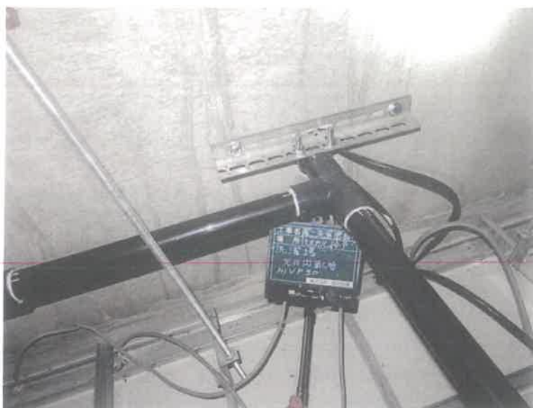
【工事種目】エスカル神戸洗濯給水配管 【施工内容1】5階洗濯室天井内 【施工内容2】配管作業H1VP30A 【施工内容3】支持金具取付 振れ留め
