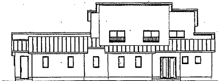
背面図 ③ 1/100
