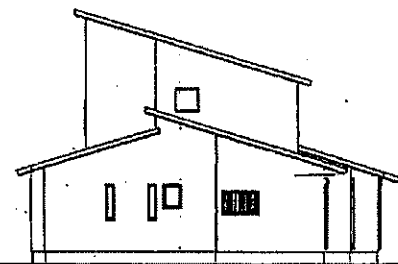
側面図 ④ 1/100
