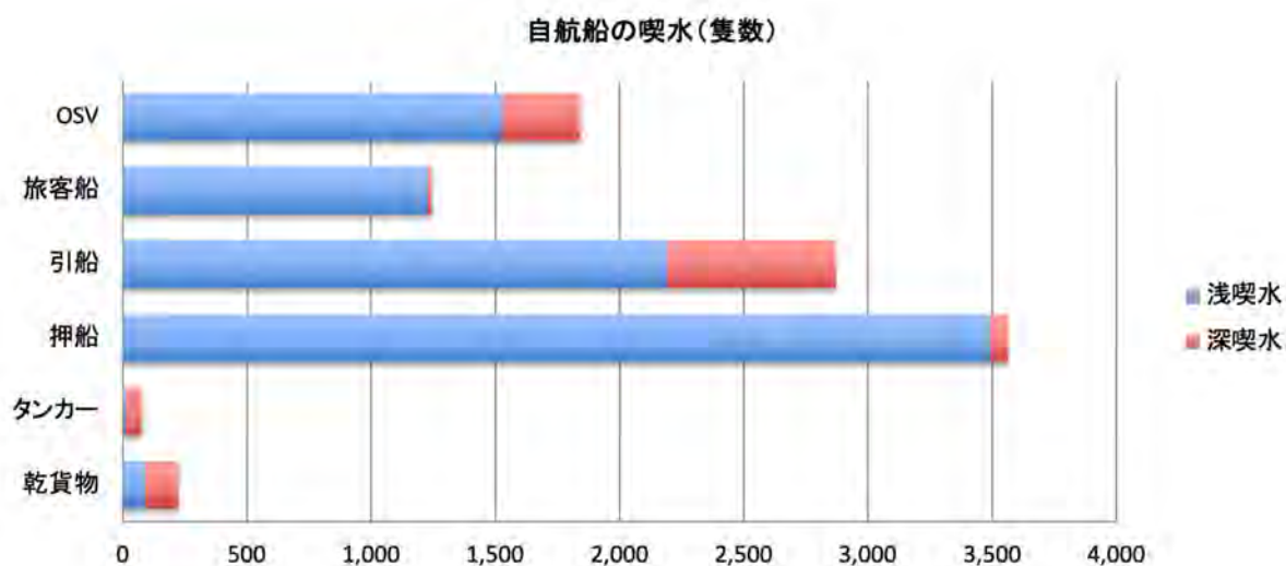
図 36 自航船の喫水（隻数）
