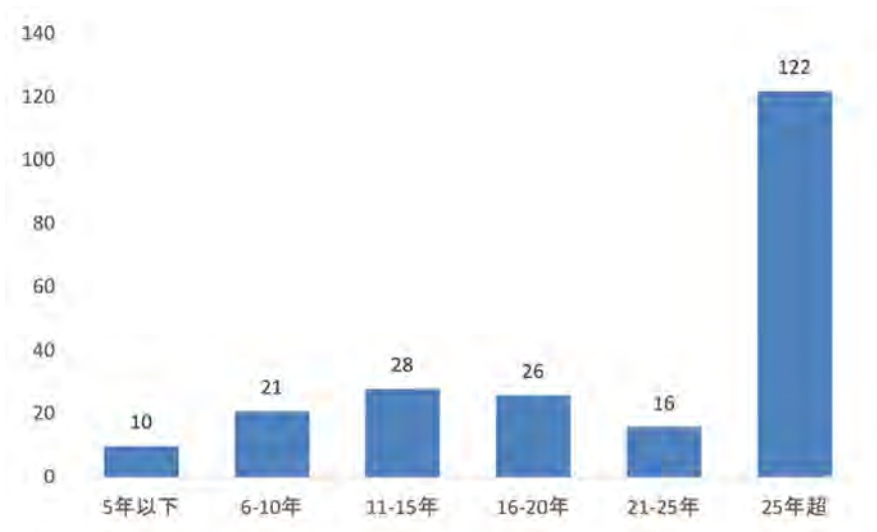
図 23 乾貨物船船齡分布（隻数）
