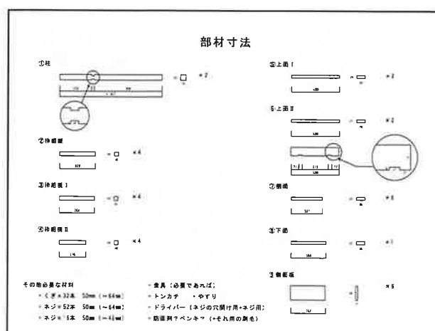
fig6. 材料表
