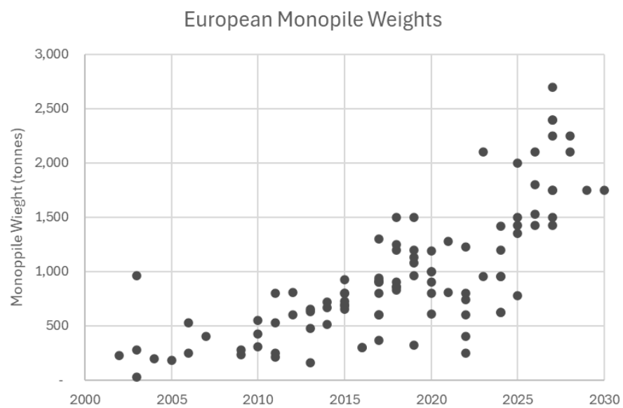
図 13 欧州プロジェクトのモノパイルの重量推移 Source; Intelatus Global Partners
