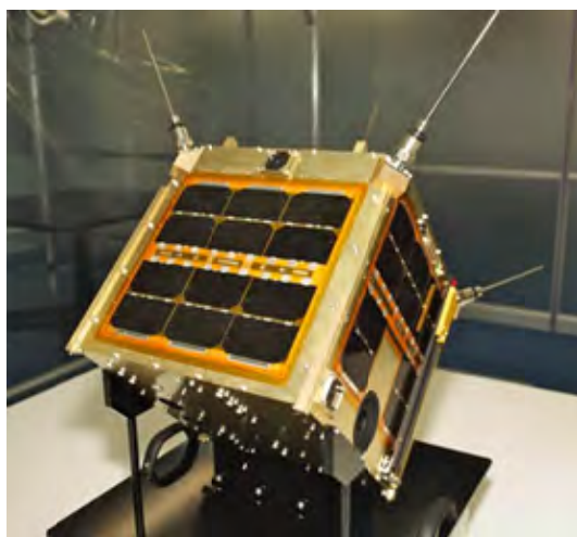
図-1.3.5 WNISAT-1
